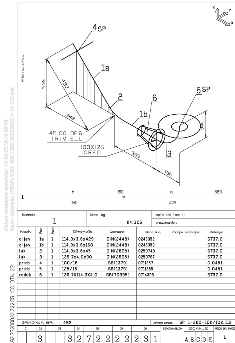
Slika 14. Mjerna skica cijevi
