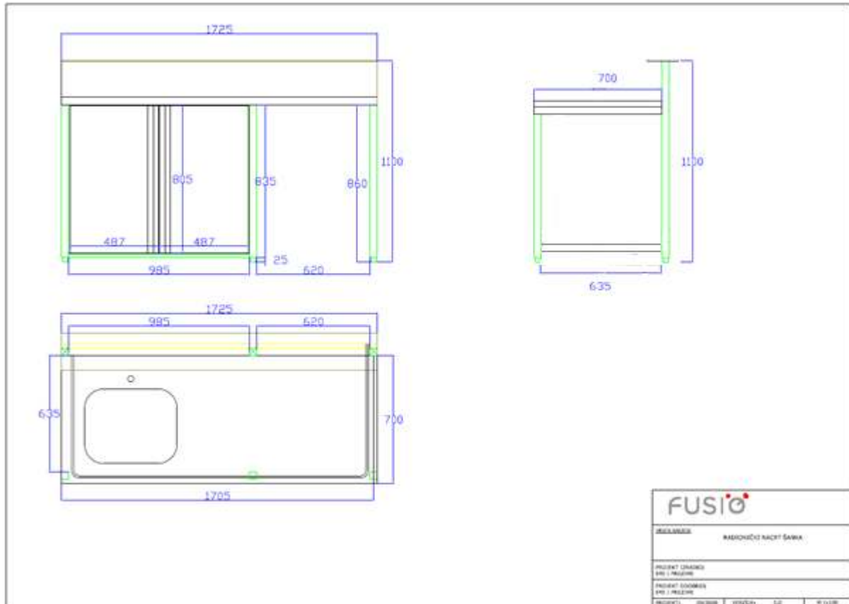
Slika 12: Radionički nacrt; Izvor:Interne slike poduzeća Fusio d.o.o.
