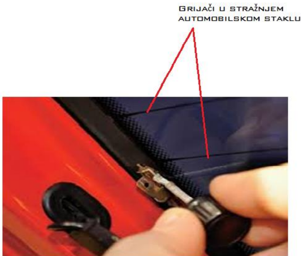
Slika 3.9. Grijači u staklu napravljeni putem sitotiska
