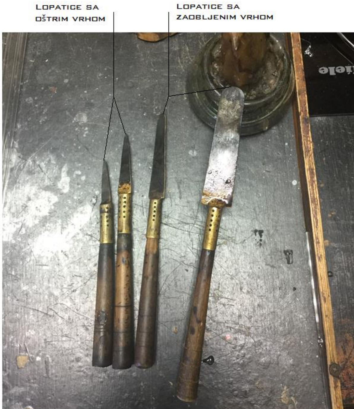
Slika 5.7. Lopatice za oblikovanje stakla
