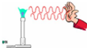
Slika 2.7. Zračenje
