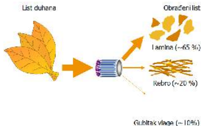
Slika 7: Obrada duhana
