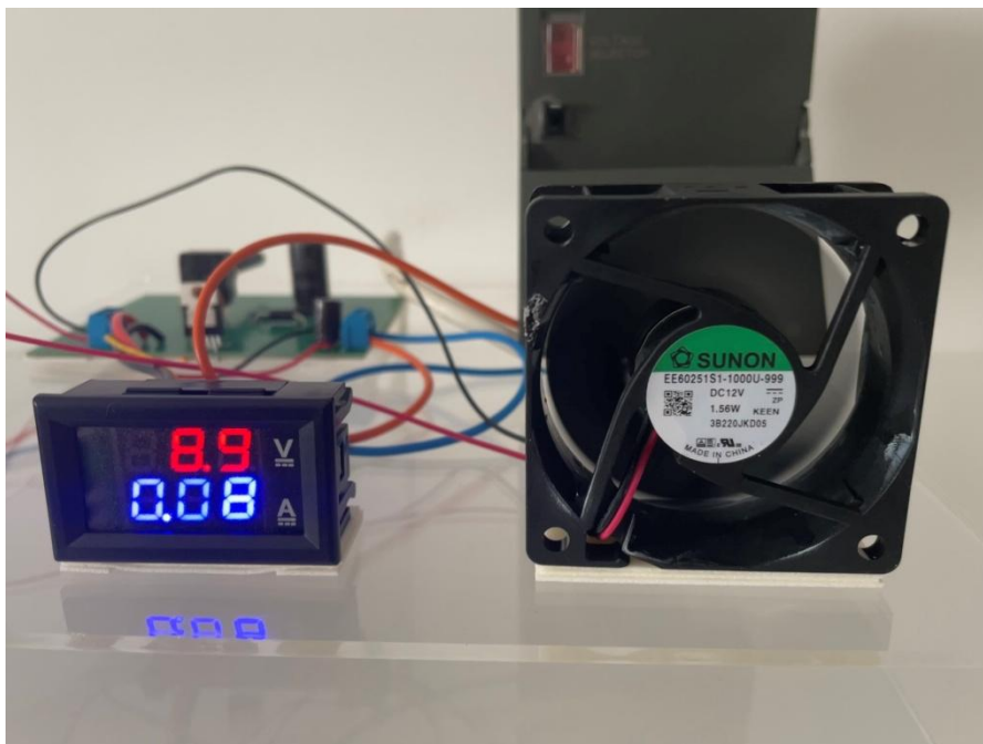
Slika 32: Izlazni napon i struja, mjerenje 3
