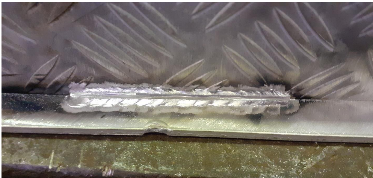
Slika 8. Prorez na zavarenom spoju
