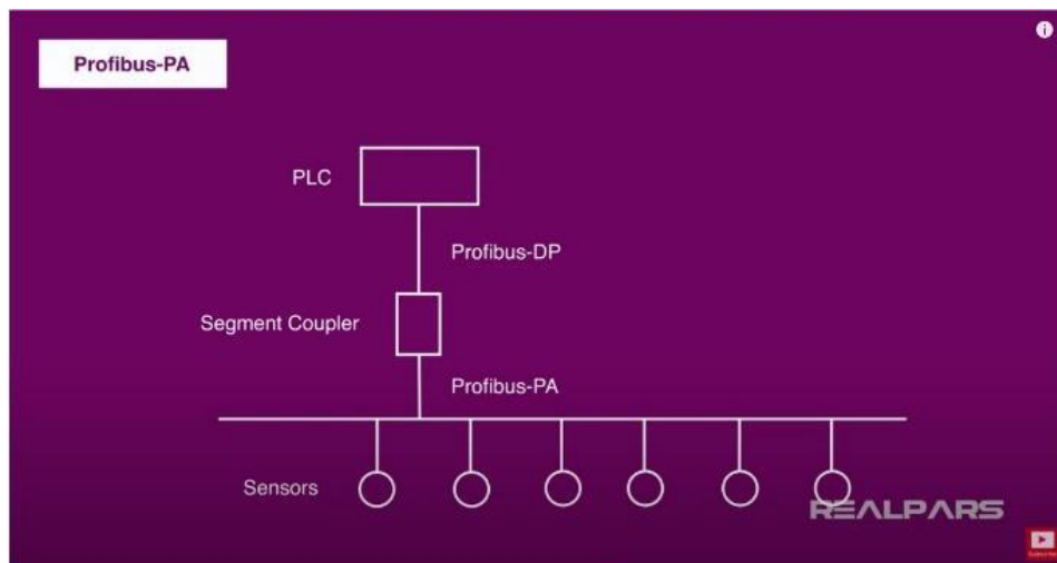
Slika 8. PROFIBUS PA
