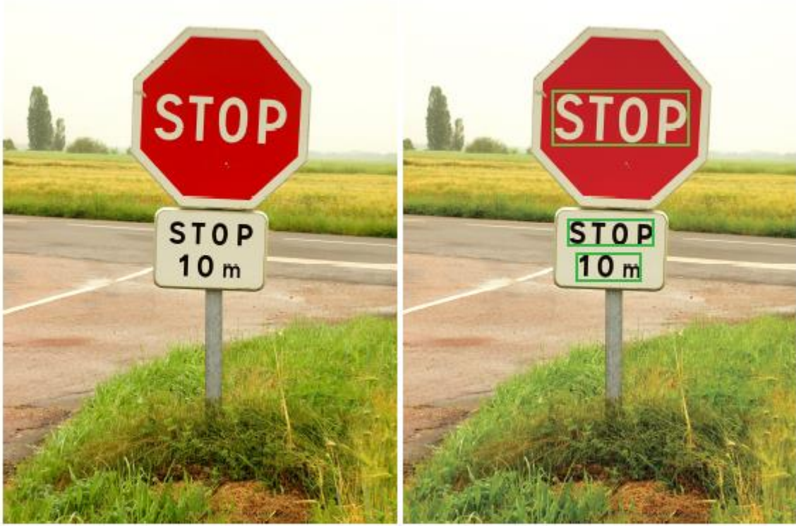
Slika 24: MSER detekcija
