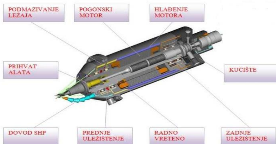
Slika 19. Motorvreteno 28
