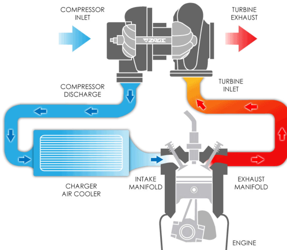
Pogon turbo punjača
