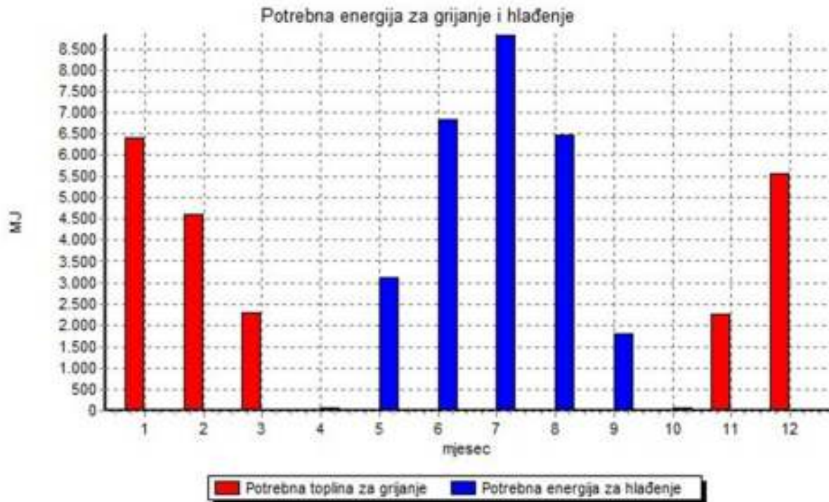
Grafikon 1. Potrebna energija za grijanje i hlađenje objekta
