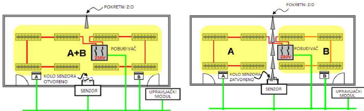
Slika 4-4 Upravljanje rasvjetom prostorije sa i bez pregrade
