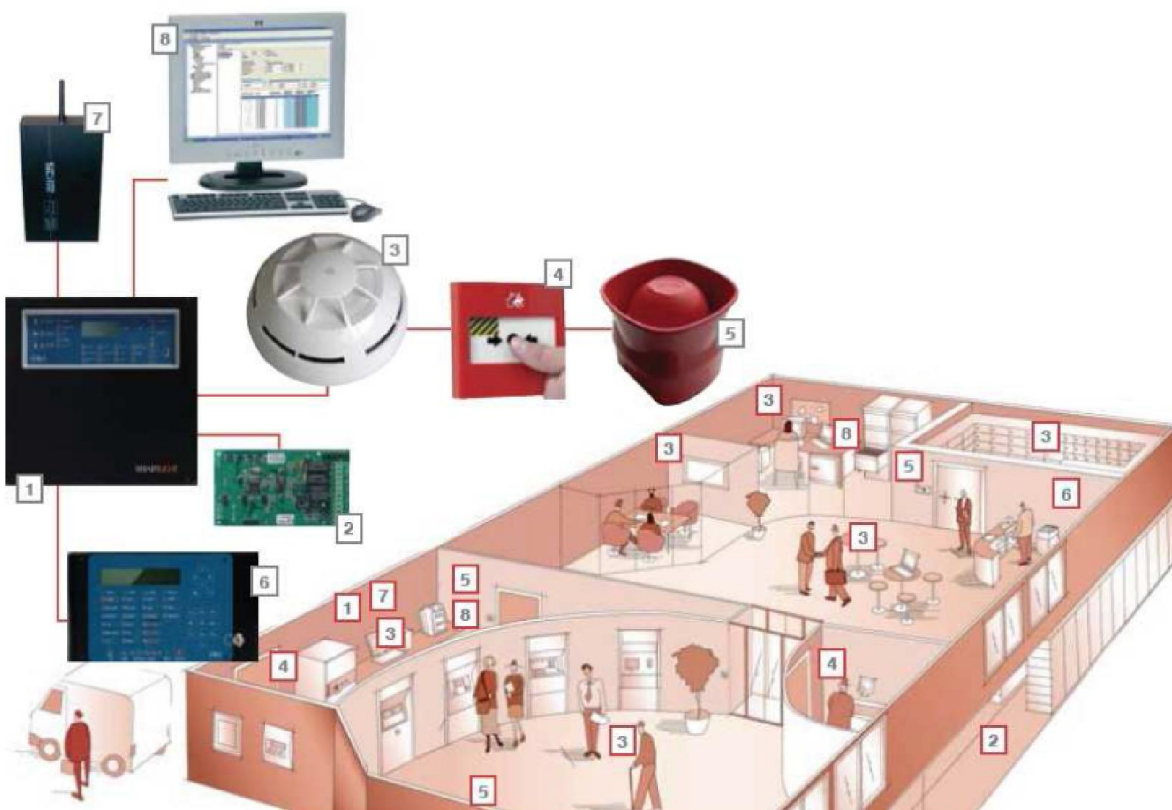
Slika 7-2 Adresabilni sustav protupožarne zaštite
