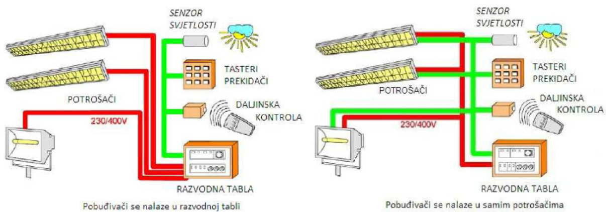
Slika 4-3 EIB instalacija
