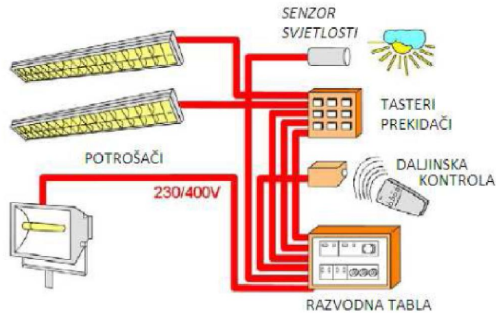
Slika 4-2 Složena instalacija u klasičnoj izvedbi
