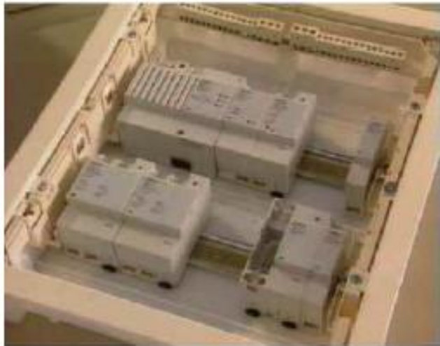
Slika 4-8 Razvodna kutija sa montiranim EIB uređajima
