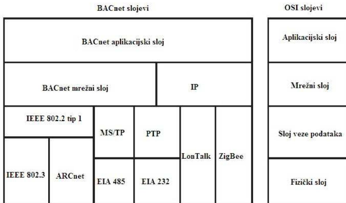
Slika 3-2 BACnet arhitektura
