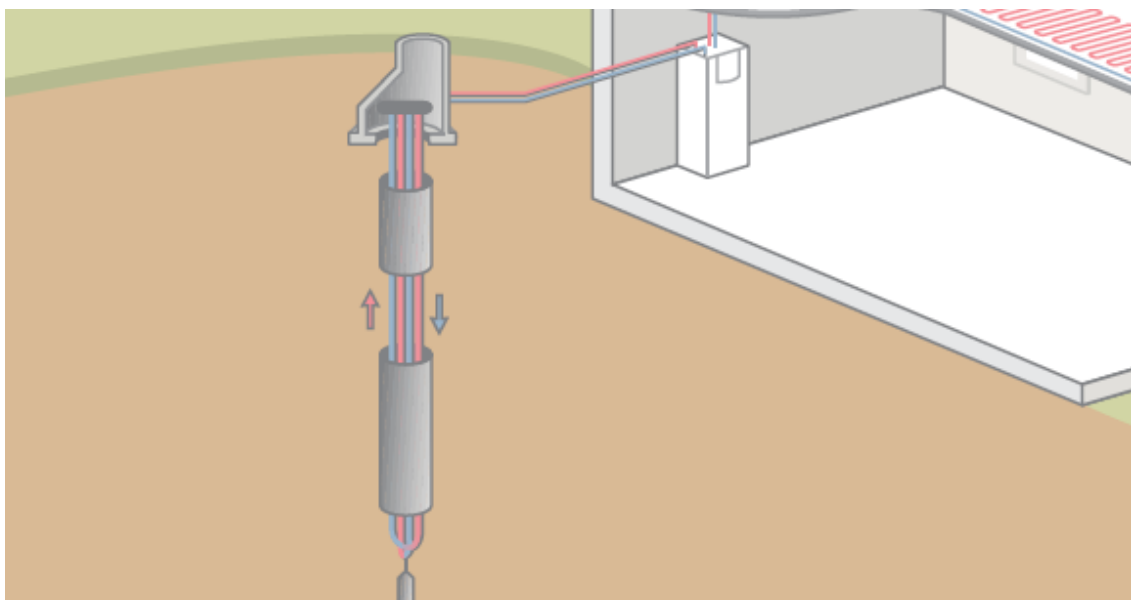
Slika 6: Dizalica topline tlo voda sa podzemnom toplinskom sondom (izvor: Prospekt Dizalice topline geoTHERM)
