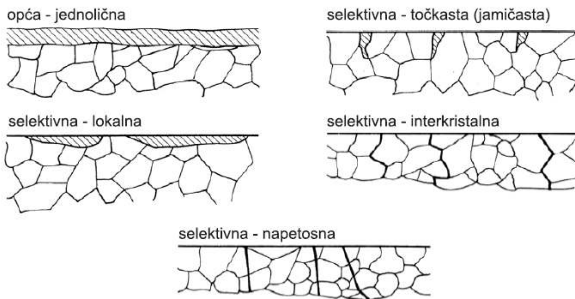
Slika 2. Shematski prikaz oblika korozije
