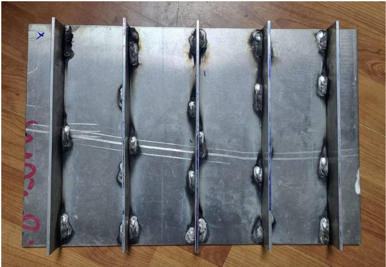
Slika 2. Pojačanja na trupu broda
