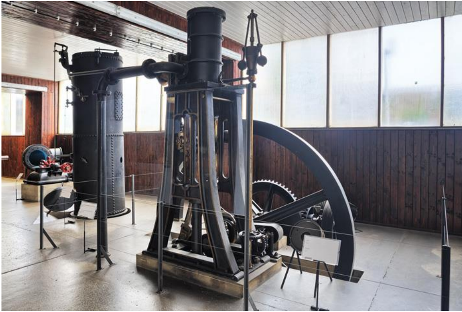
Slika 1: Parni stroj
