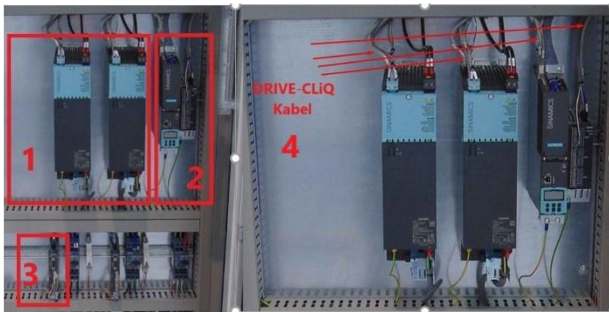
Slika 16. Praktičan primjer Siemens Sinamics S120 modularni sustava i CU320-2 (izvor: autor, 11.8.2021.)
