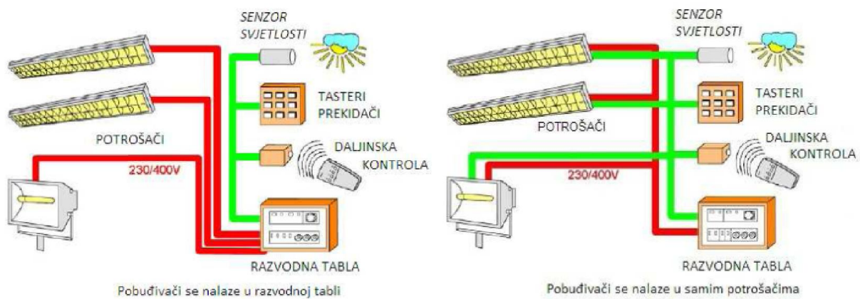
Slika 4-3 EIB instalacija
