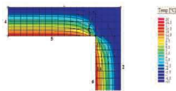
Slika 10. Prikaz toplinskog mosta na izoliranom kutu zgrade
