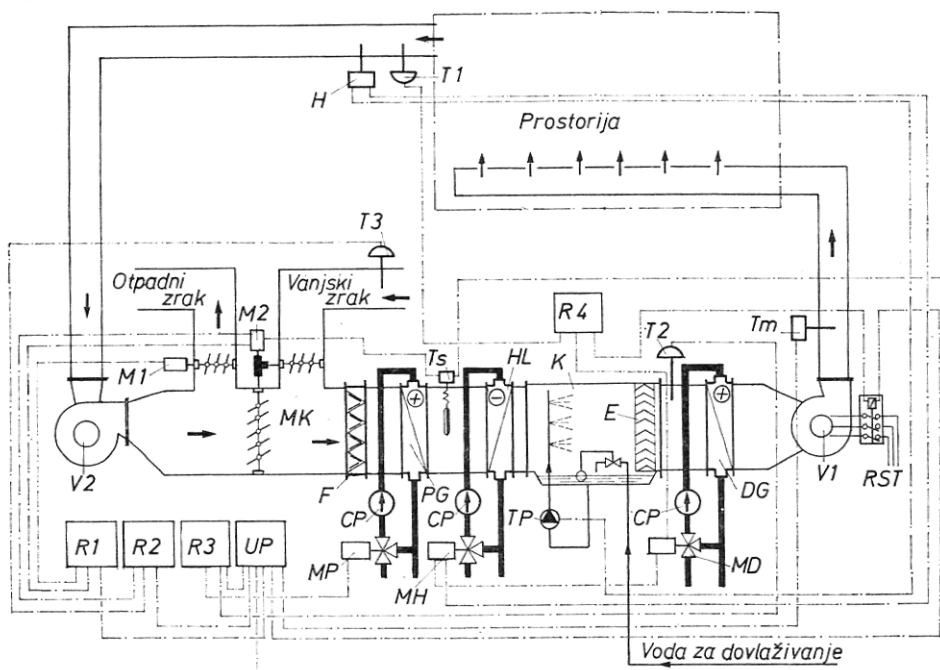
Slika 25. Shema postrojenja za klimatizaciju
