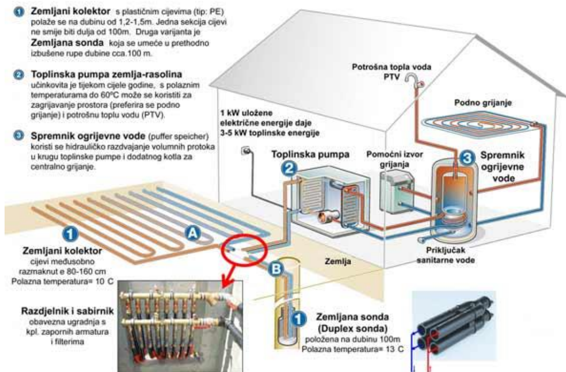
Slika 5: Način izvođenja i dijelovi za izvođenje dizalice topline sa zemljanim kolektorom (izvor: Propekt Dizalice topline geoTHERM)
