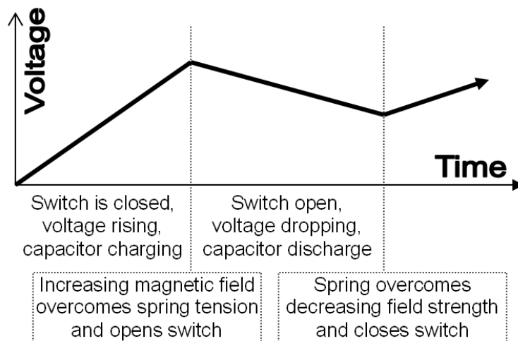
Slika 1: Grafikon izlaznog napona na vremenskoj skali
