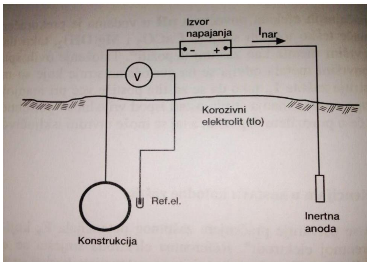
Slika 12. Dijagramski prikaz sustava katodne zaštite narinutom strujom
