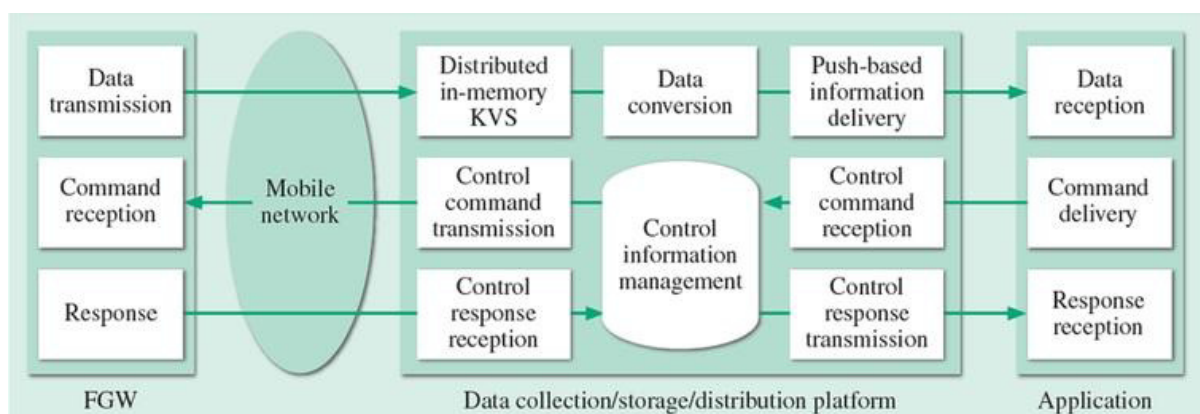
Slika 25: Prikaz Hitachi sustava za "tvornice biljaka"
