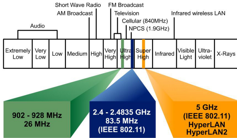
Slika 12: Radiofrekvencijski spektar
