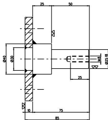
55 N°1 PEZZO - Acc. INOX AISI 304
