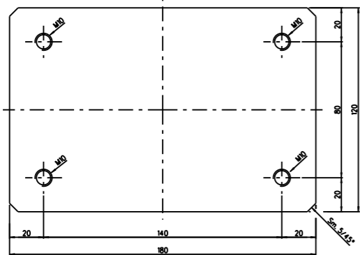
12 N°1 PEZZO - Acc. INOX AISI 304
