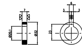
71 N°1 PEZZO - Acc. INOX AISI 304
