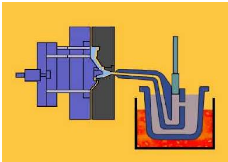
Slika 11. Shema tlačnog lijevanja s toplom komorom [11]
