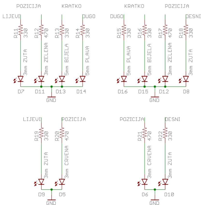
Slika 23. Električni spoj LED dioda i otpornika „BDM“ modula
