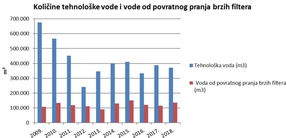
Slika 35: Grafički prikaz količine tehnološke vode i vode od povratnog pranja brzih filtera u periodu od 2009. do 2018. godine [Autor]
