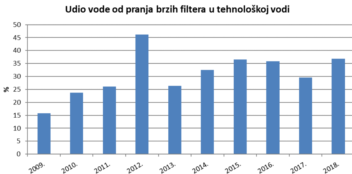
Slika 36: Grafički prikaz udjela vode od povratnog pranja filtera u tehnološkoj vodi u periodu od 2009. do 2018. godine [Autor]
