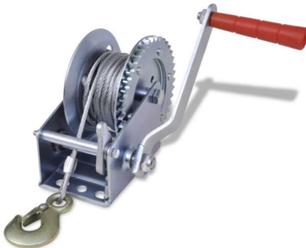
Slika 2. Ručno vitlo
