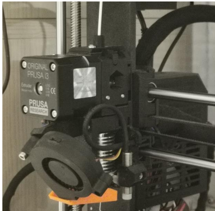
Slika 62. Ekstruder
